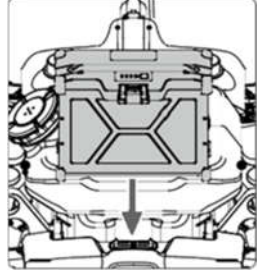
Akıllı Uçuş Bataryasını bir tık sesi duyana kadar yuvasına yerleştirin.
